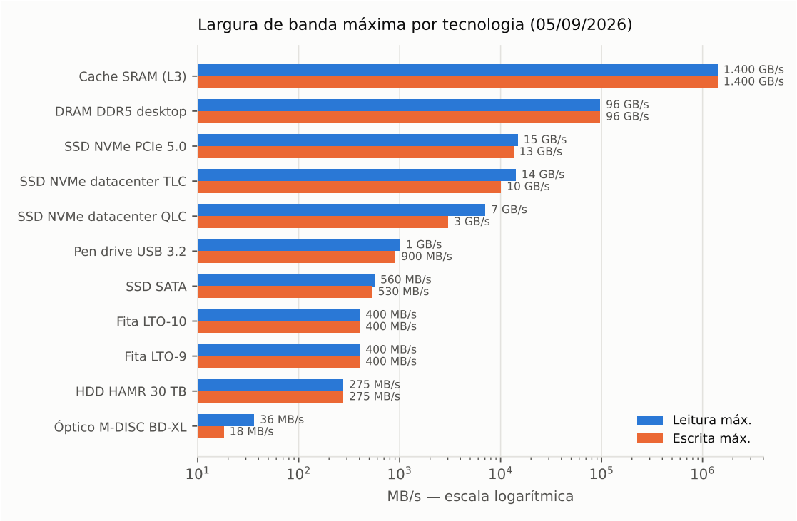
Figura 2: Largura de banda de leitura e escrita por tecnologia (escala logarítmica). O SSD NVMe PCIe 5.0 entrega 20× a banda da Tabela 16.1 original para SSD (750 MB/s → 14,7 GB/s), enquanto o disco magnético avançou apenas 1,4×. Note que a fita LTO ultrapassa o disco magnético em taxa sequencial — fato contraintuitivo que decorre de a fita não precisar posicionar um braço entre blocos consecutivos.
